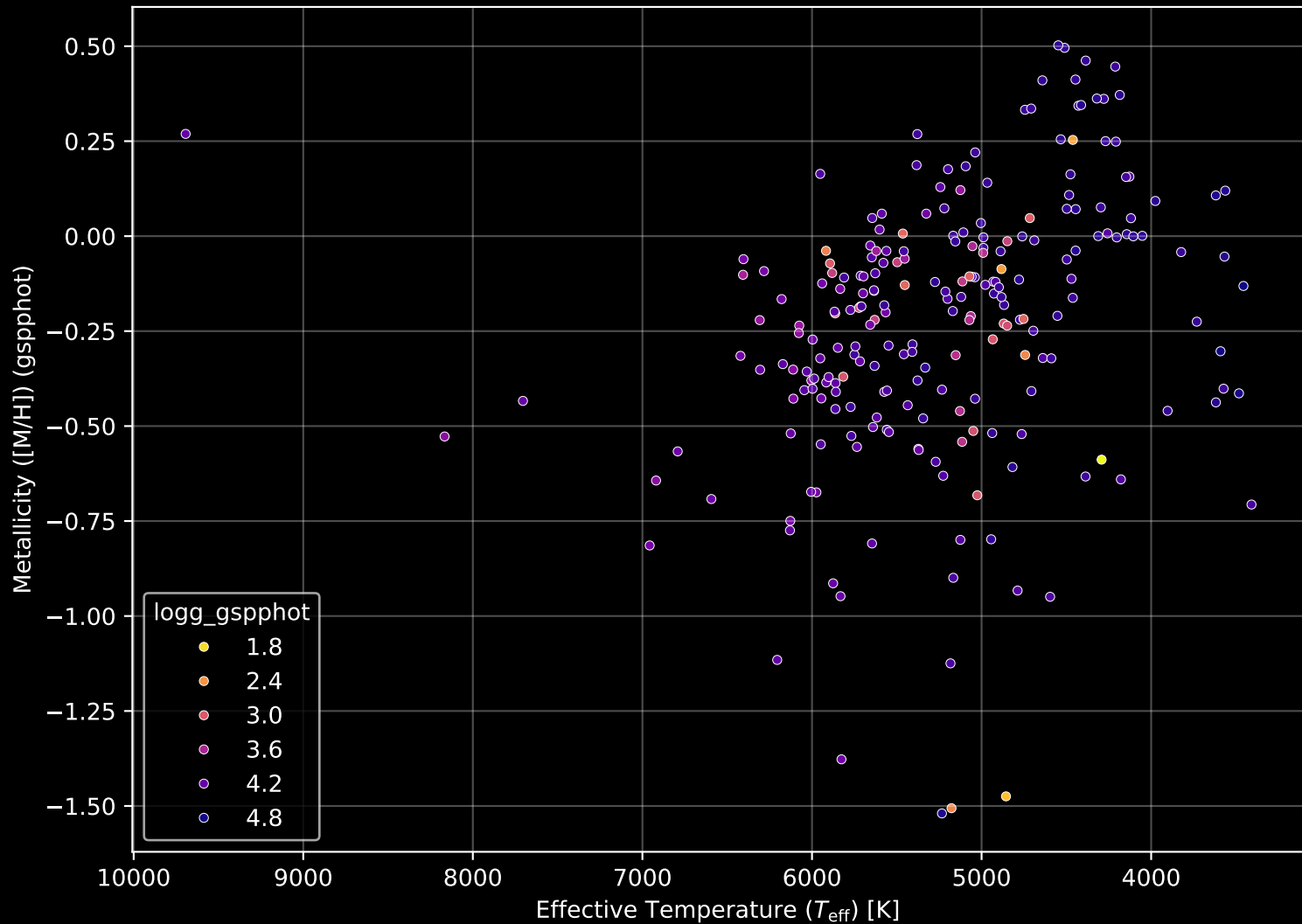
APOGEE DR17 Field: [232+66_btx] Stellar Population Parameters (n= 230)
